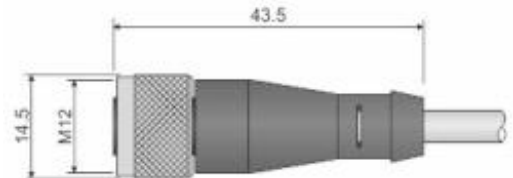
Connettore femmina M12 - versione dritta M12 female connector - straight type
